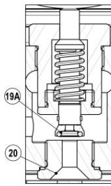
Detalhe A Válvula piloto (suave)
