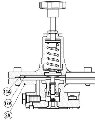
Parte superior de baixa pressão
