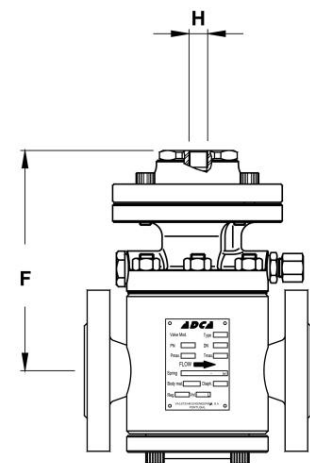
Fig. 3 - Válvula carregada em cúpula
