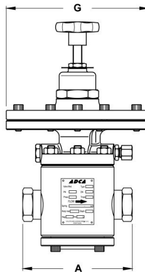
Fig. 1 - Válvula com diafragma padrão
