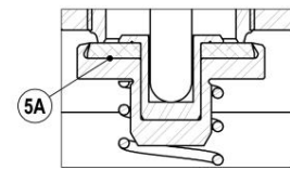
Detalhe B Válvula principal (suave)
