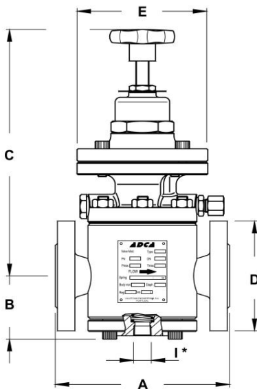
Fig. 1 - Válvula com diafragma padrão
