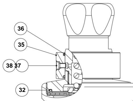
Conexão de linha de vazamento opcional
