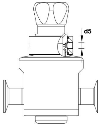
Conexão de linha de vazamento opcional
