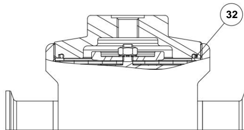
Carregamento de cúpula opcional
