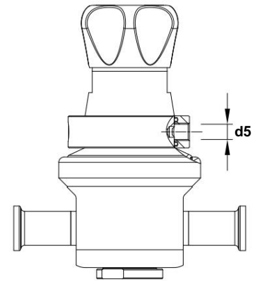
Conexão de linha de vazamento opcional
