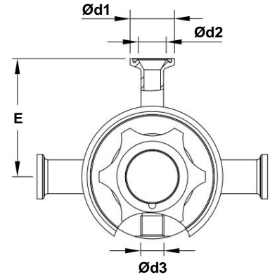
Conexão de medidor opcional
