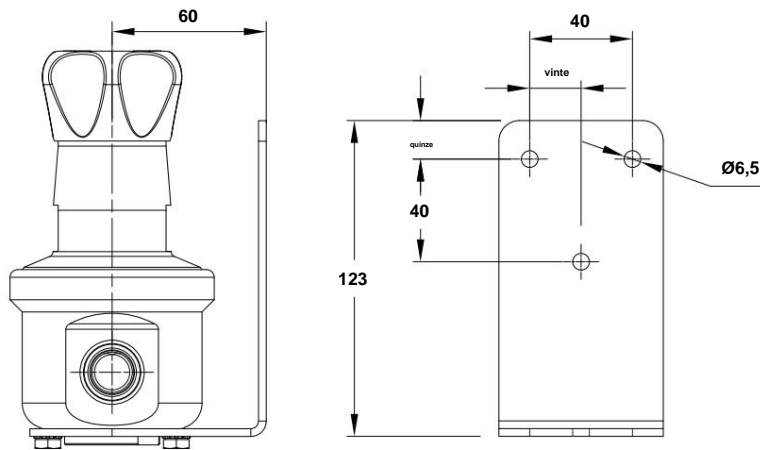
Montagem na parede opcional
