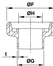
DIN 11851
