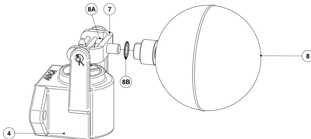
Fig. 5 - Substituição da bóia.
