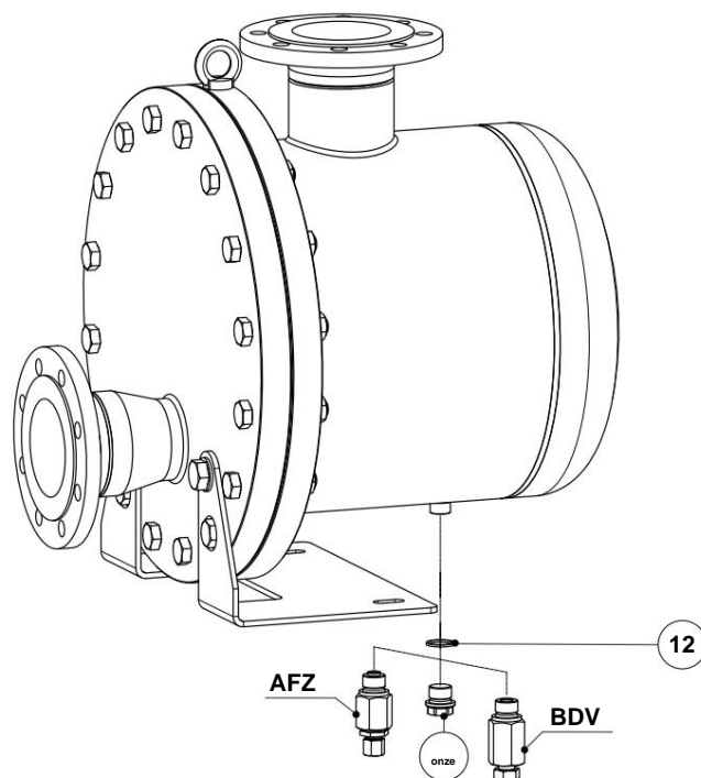
Fig. 6 - Unidades opcionais BDV e AFZ.
