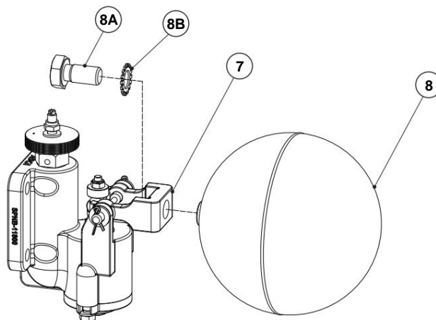
Fig. 7 - Substituição da bóia.
